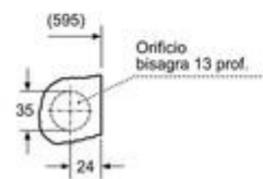
Detalle Z
