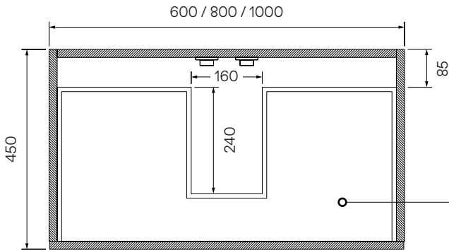
Vista superior
