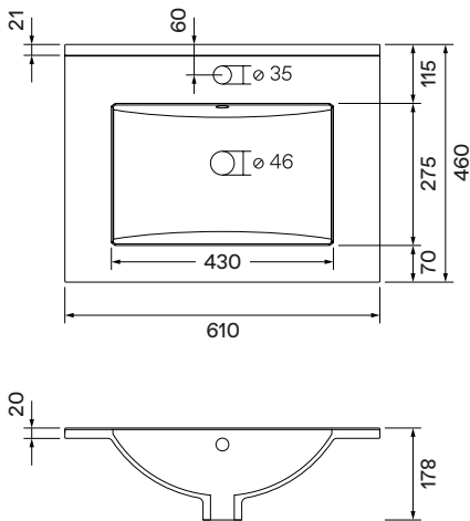
Cerámico 60
