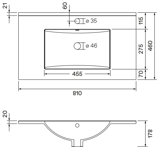
Cerámico 80
