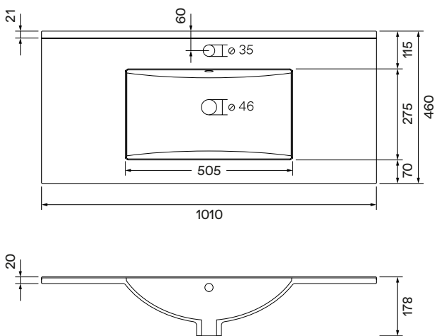
Cerámico 100
