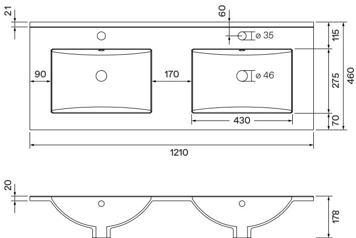
Cerámico 120
