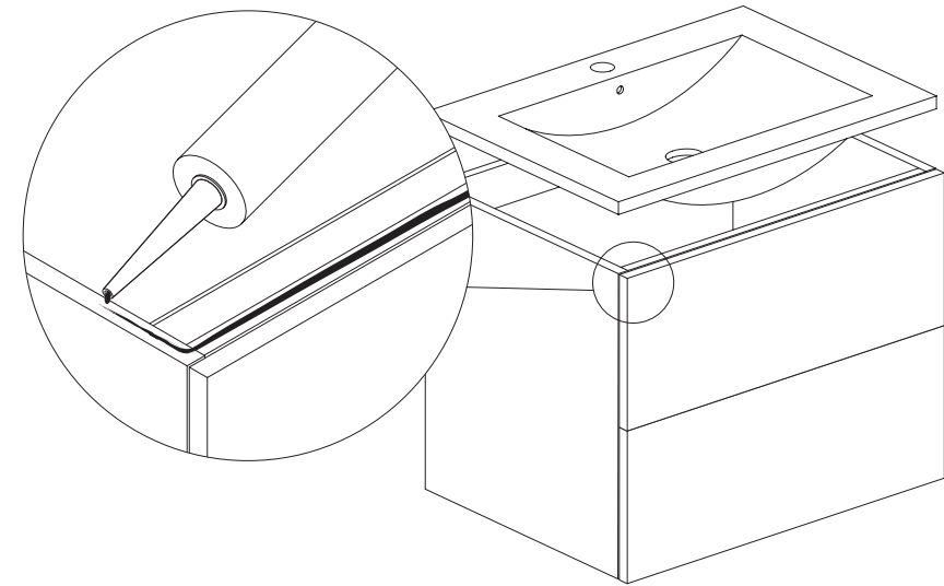
Typ 2. Aufsatzwaschbecken
