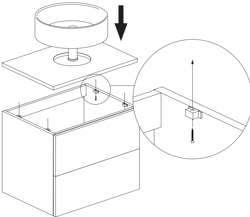
Typ 2. Aufsatzwaschbecken
